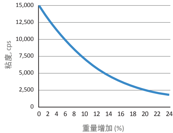
NC-513与Ultra LITE 513稀释曲线图 (25°C/与液体环氧混合, 环氧当量=190)
