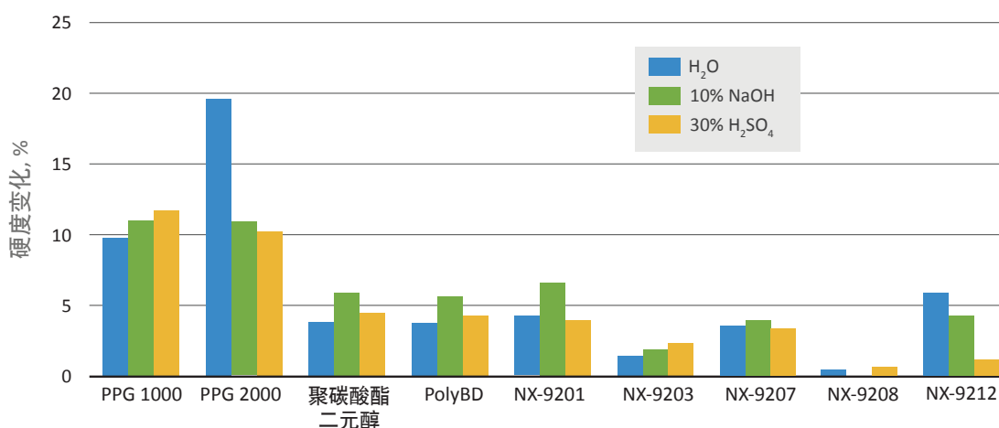
二元醇的水解稳定性 *固化的预聚体 (7% NCO): 21天/25°C测试
