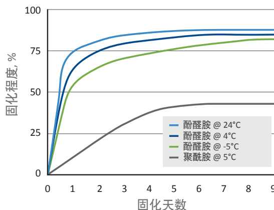
酚醛胺低温固化数据及对比
