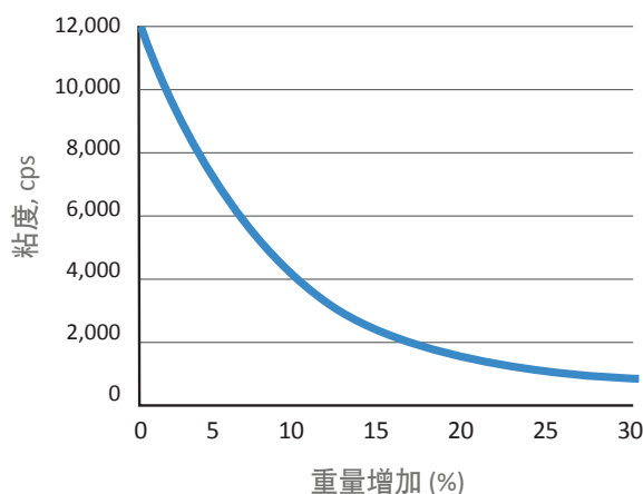
NX-202x与LITE/UL 2020稀释曲线 (25°C，与液体环氧树脂混合, EEW=190)
