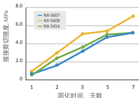
与液体环氧的粘接强度发展(环氧当量190) 基材: 喷砂钢板, 温度: 0°C
